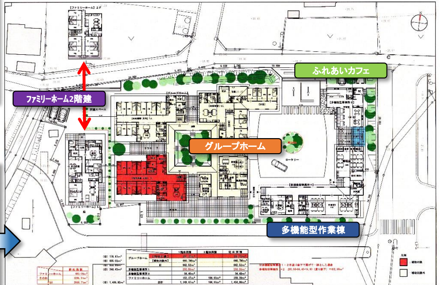
【障がい者グループホーム他 計画平面図】
